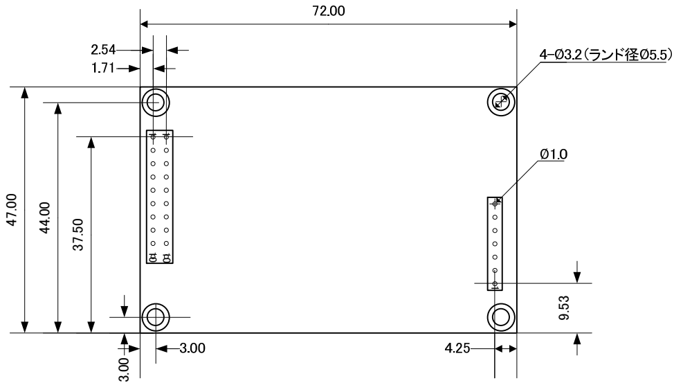
図 4.1. 基板寸法図
