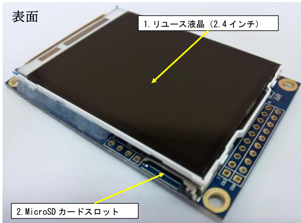
図 3.1. e-DISP3 全体図
